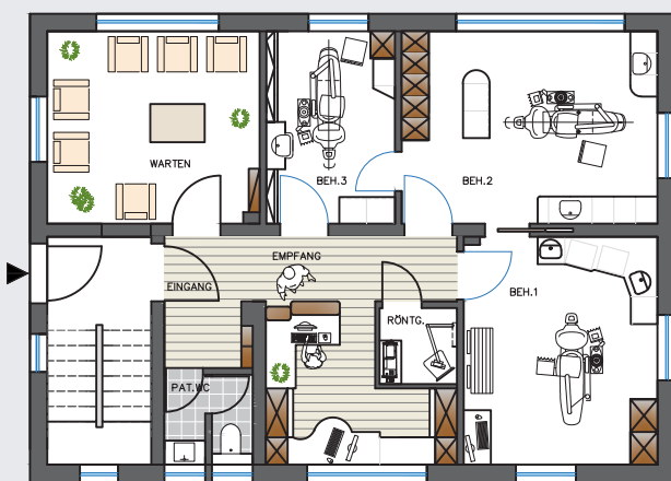
ERDGESCHOSS
